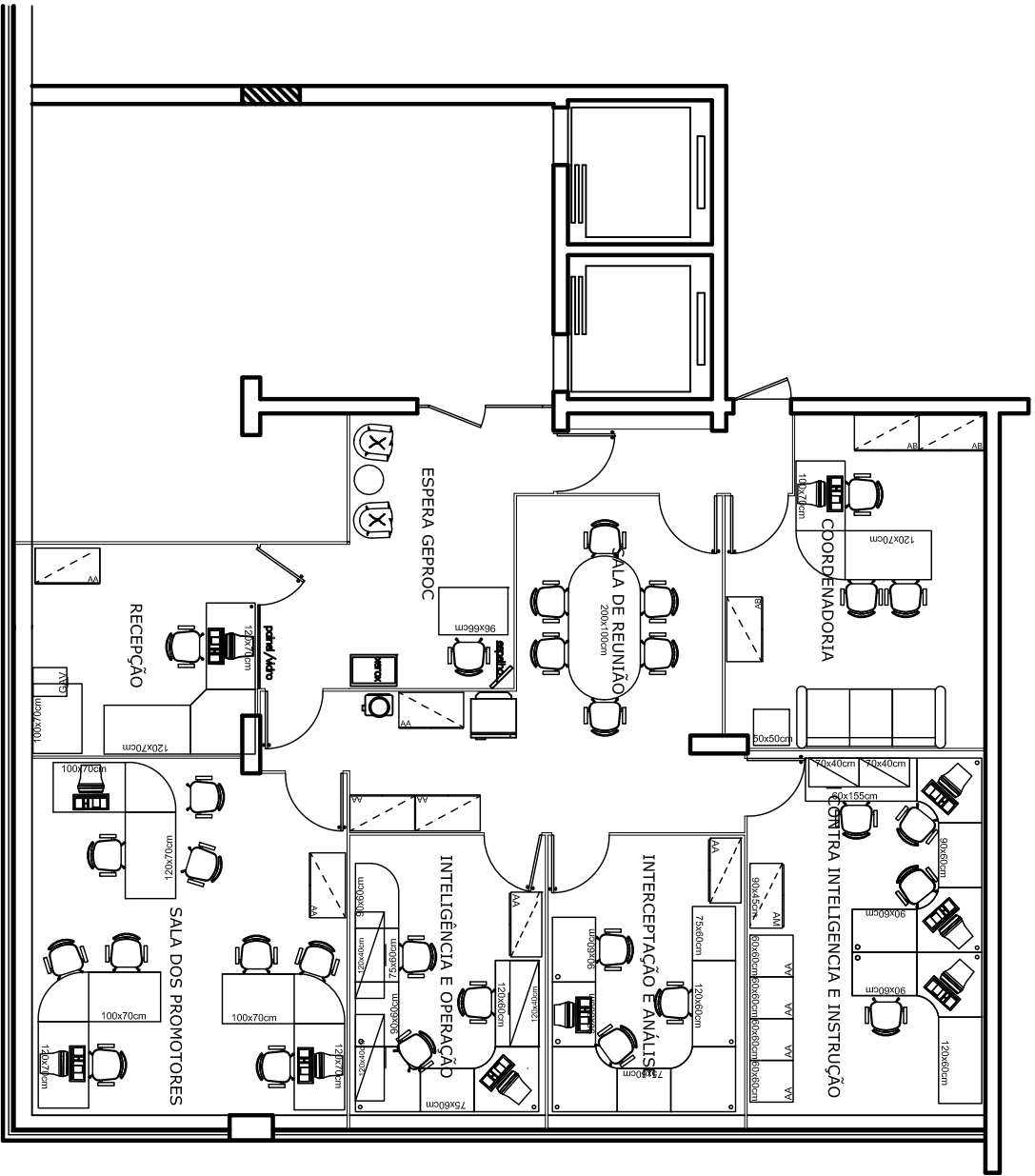
LAYOUT 4º PAVIMENTO - GEPROC Nova Proposta - junho/2011 ESC: 1/100
