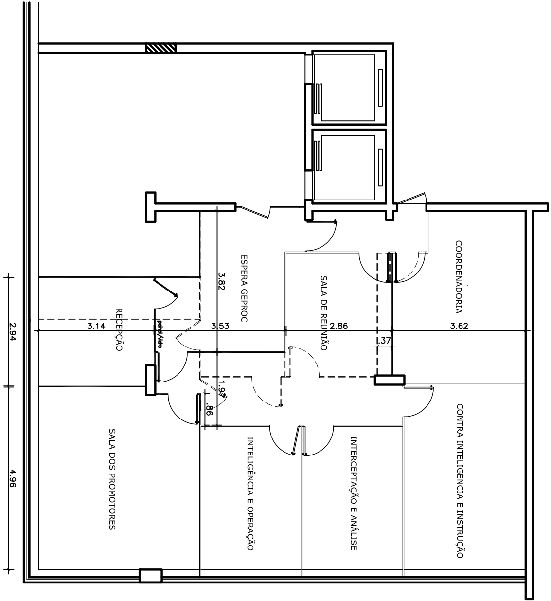
4º PAVIMENTO - GEPROC Nova Proposta - junho/2011 ESC: 1/100
