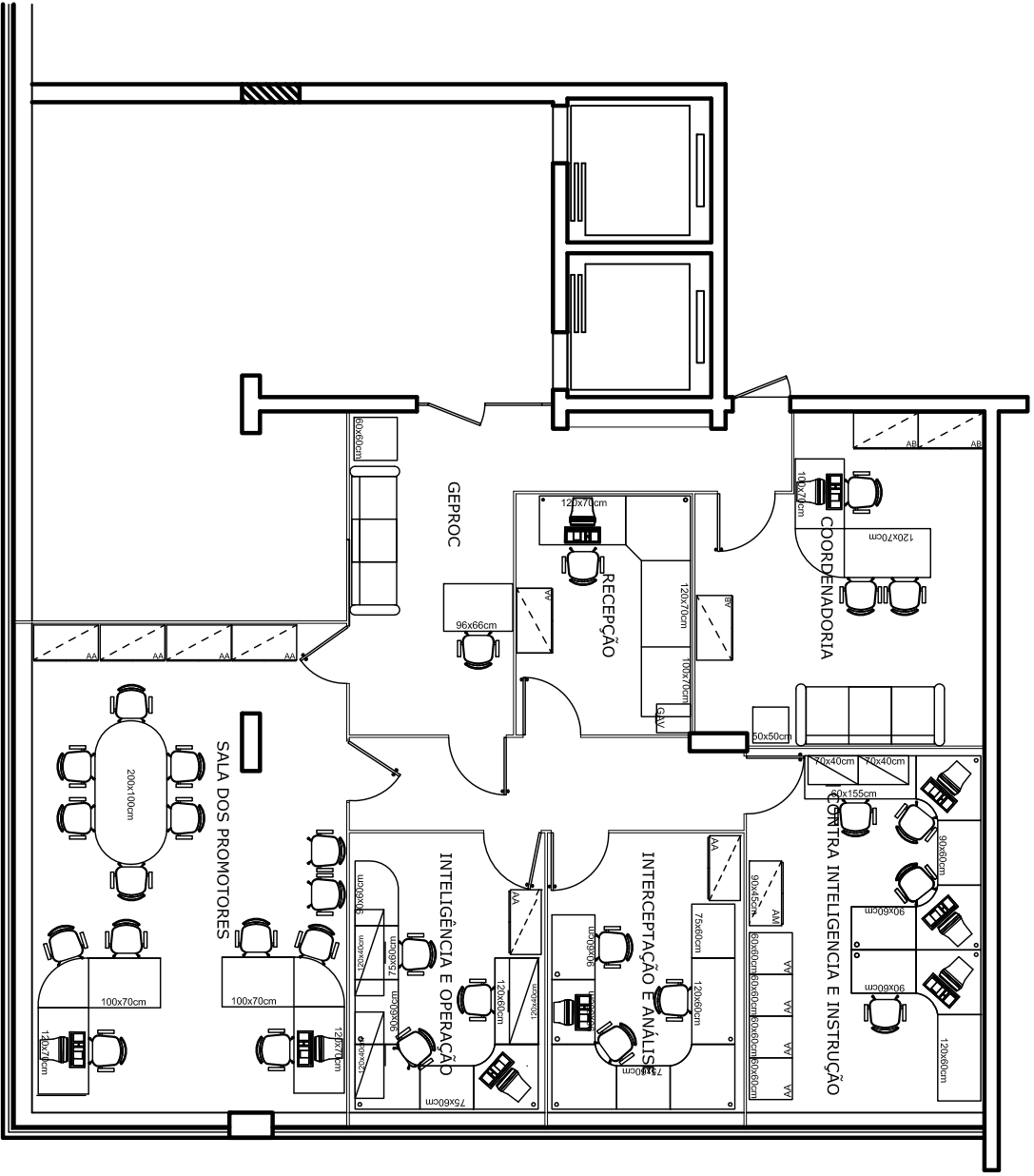
LAYOUT 4º PAVIMENTO levantamento ESC: 1/100
